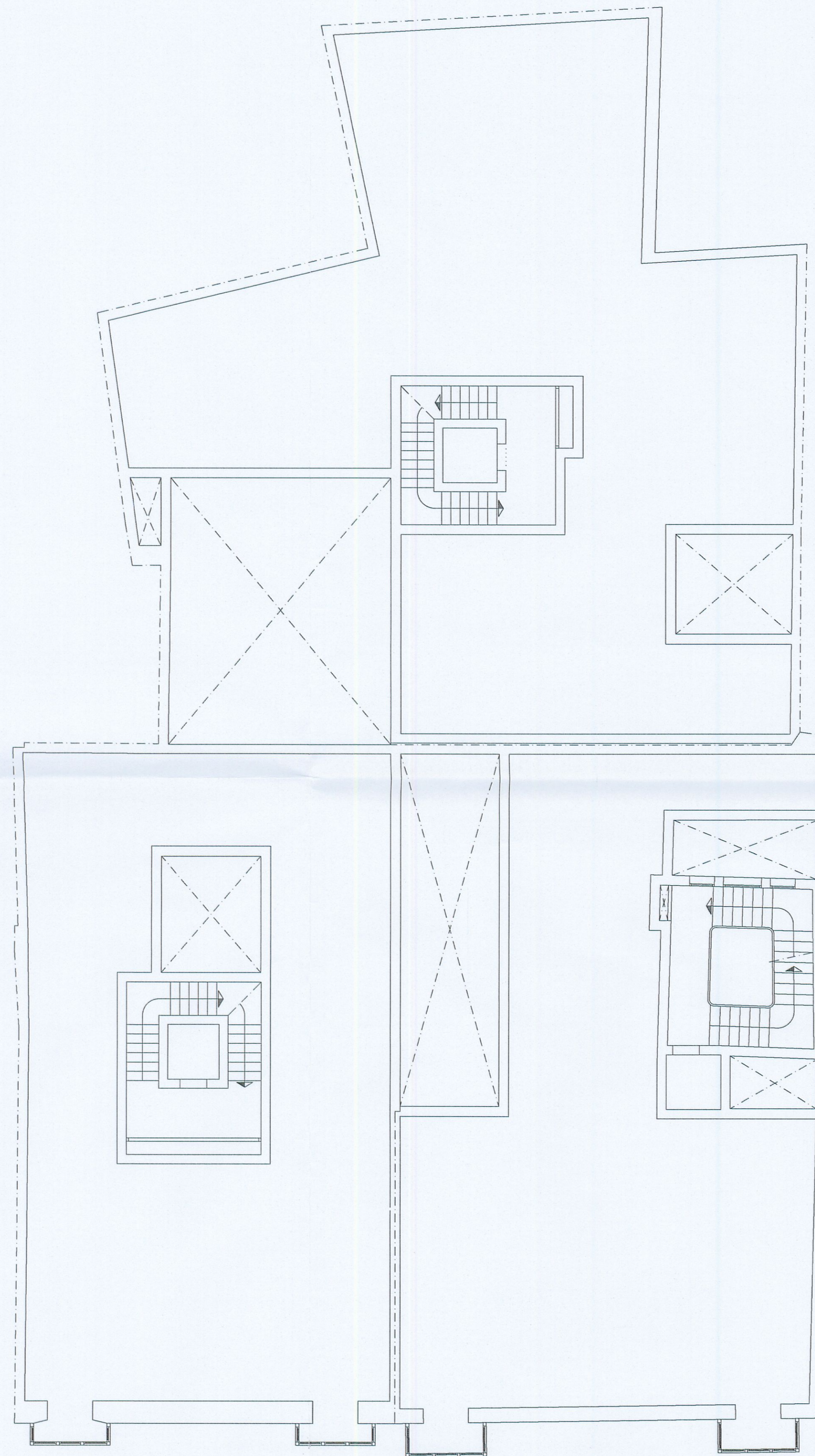
PLANTAS PISO 1 Y 2.- SUPERFICIE CONST.: 747,00 x 2 = 1.494,00 m2
