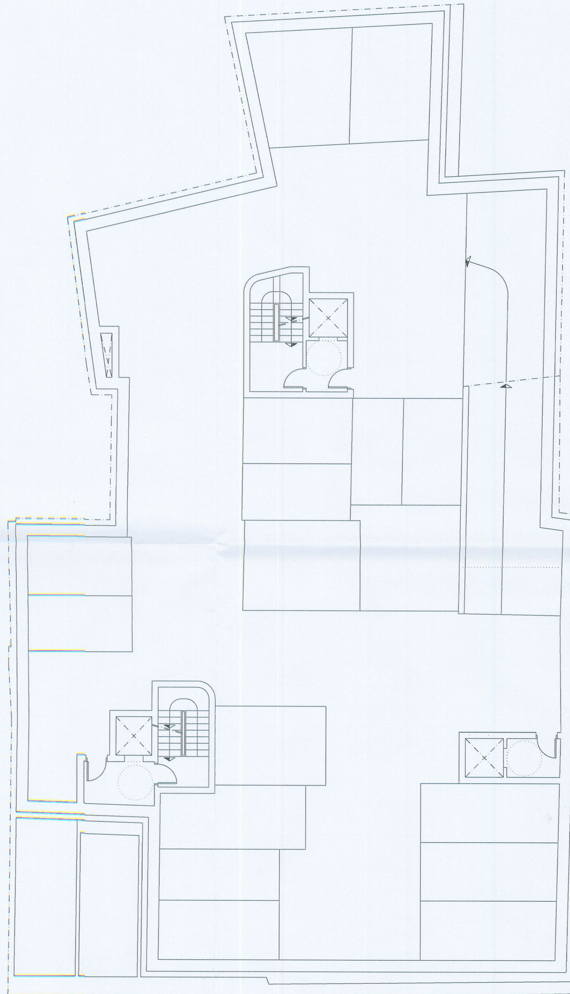
PLANTA SOTANO 1.- SUPERFICIE CONST.: 759,42 m2
