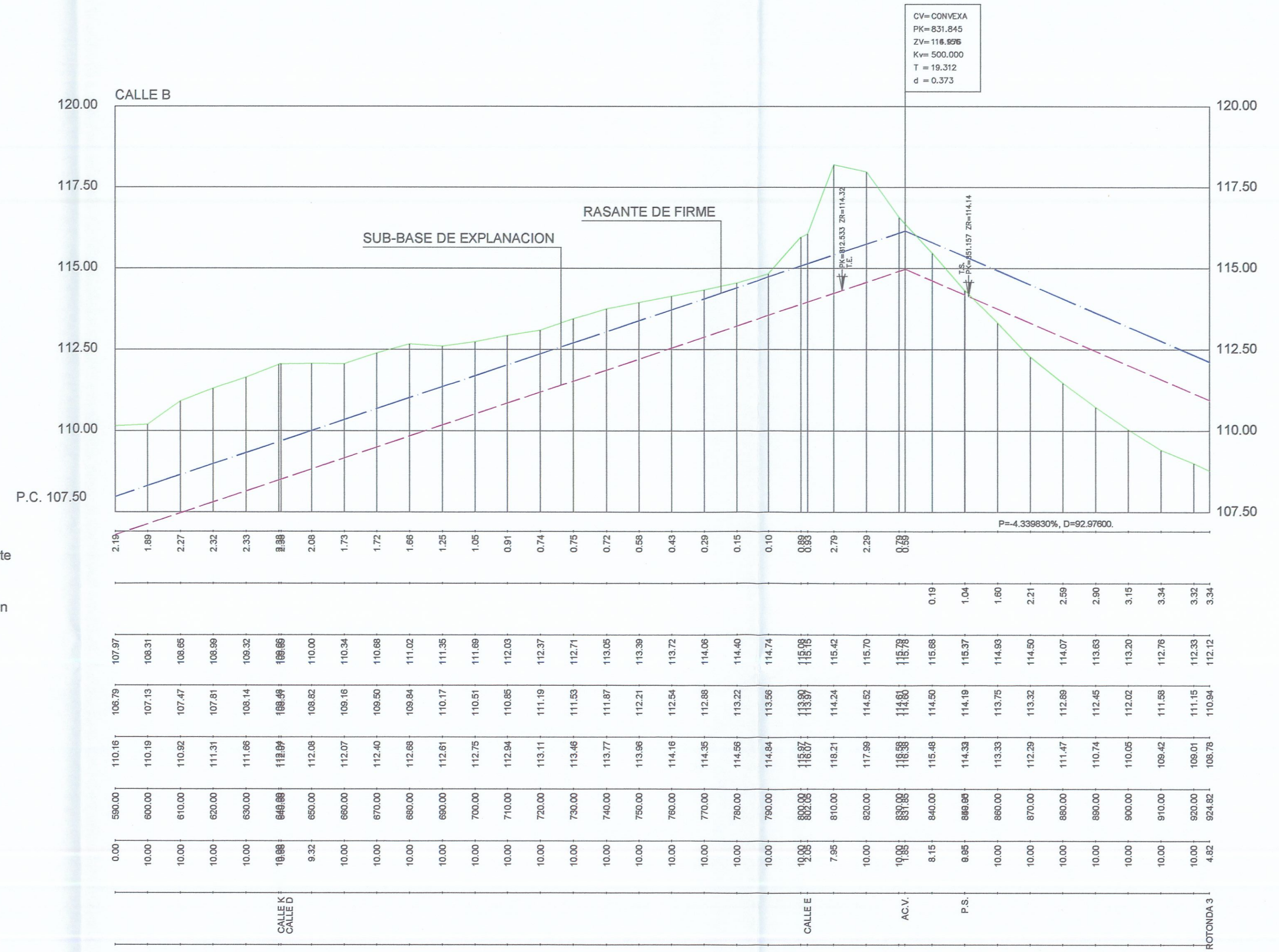
PERFIL LONGITUDINAL CALLE B
