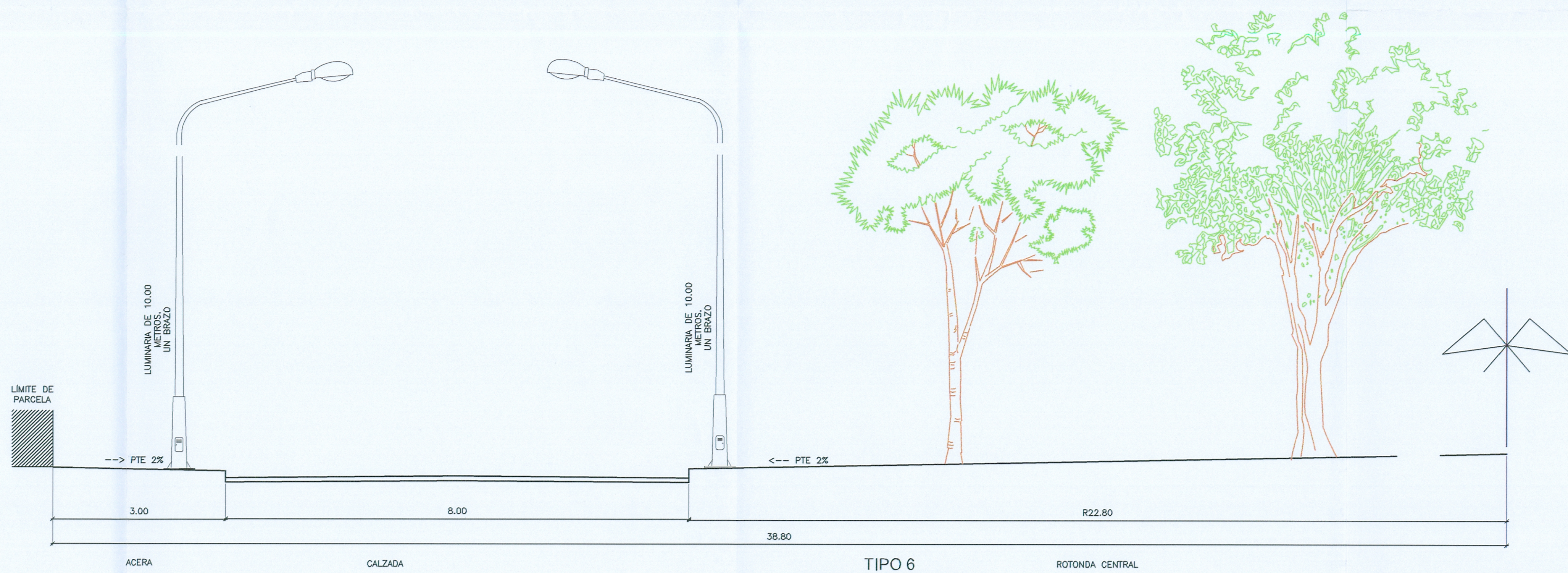
TIPO 6 SECCIÓN TRANSVERSAL VIAL DE R33,83 METROS
