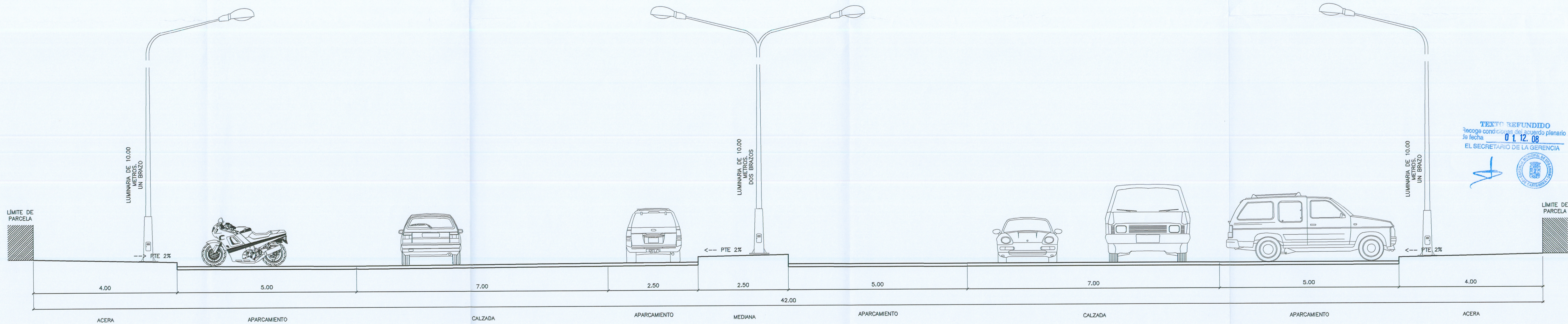
TIPO 1.2 SECCIÓN TRANSVERSAL VIAL DE 42,00 METROS
