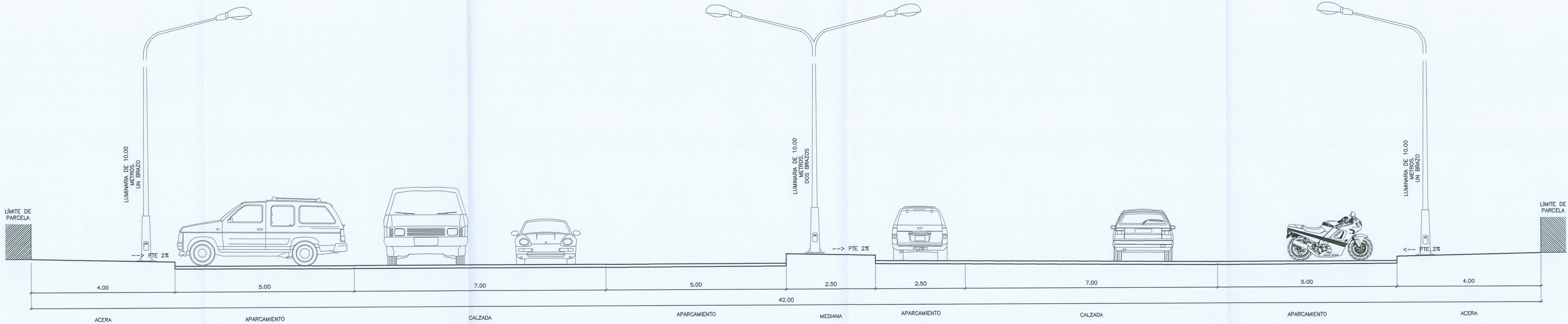
TIPO 1.1 SECCIÓN TRANSVERSAL VIAL DE 42,00 METROS
