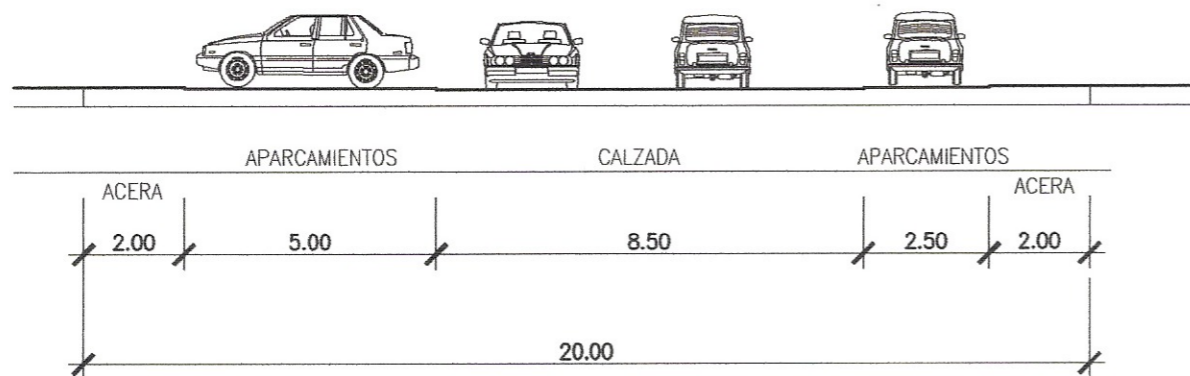
SECCION TRANSVERSAL B-B'
